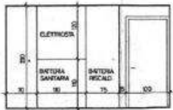
VISTA B-B
