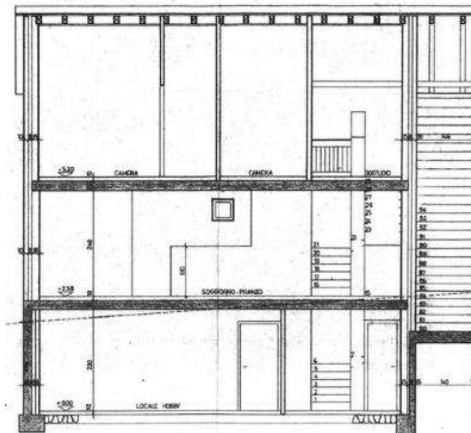
SEZIONE F.F.
